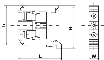
Рис. 1. Габаритные размеры зажимов наборных серии ЗН-101
